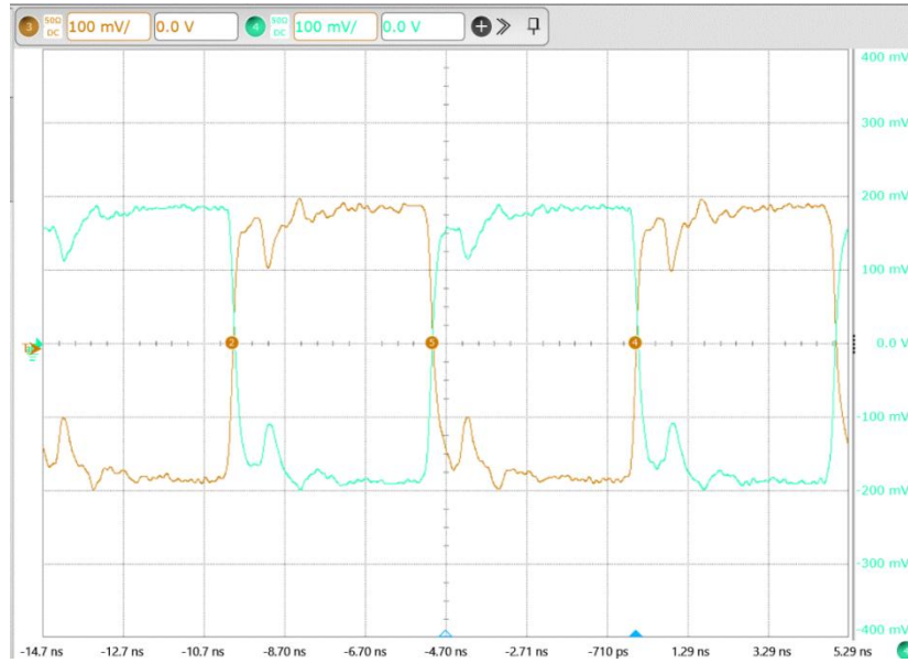
图 MBUFLVD2108 100MHz输出信号波形
