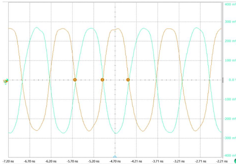
图 MBUFLVD2108 800MHz输出信号波形
