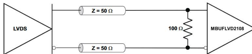
图 LVDS时钟驱动器连接到MBUFLVD2108输入（DC耦合）
