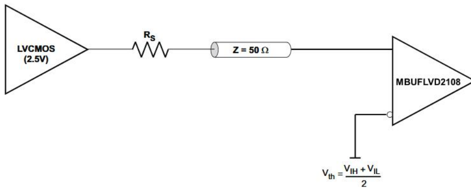
图 2.5 V LVCMOS时钟驱动器连接到MBUFLVD2108输入
