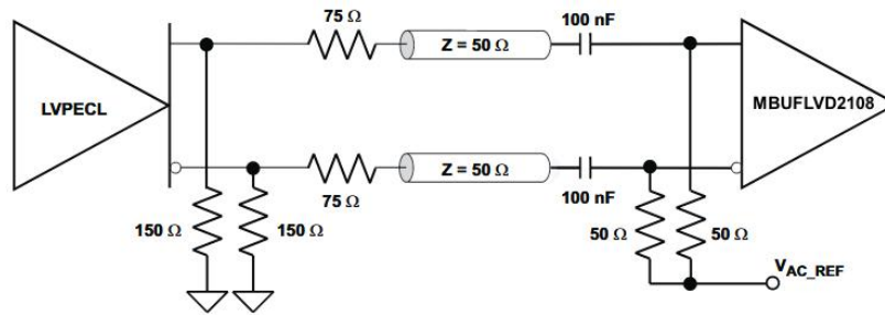
图 LVPECL时钟驱动器连接到MBUFLVD2108输入
