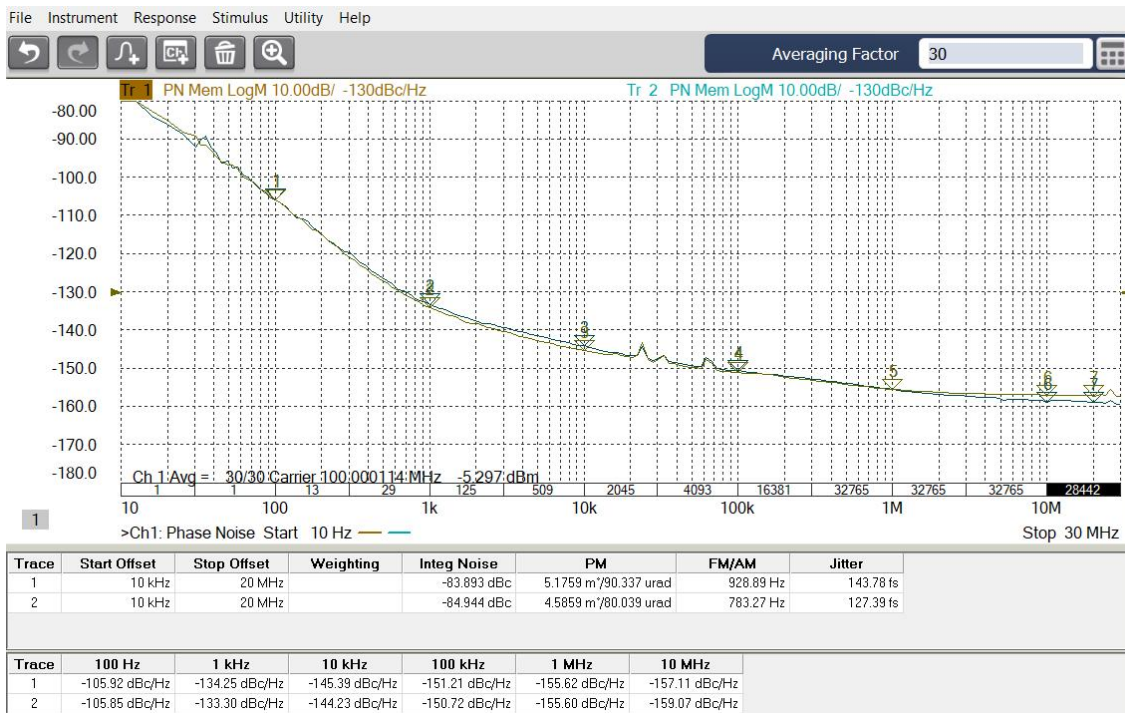
图 MBUFLVD2108在100MHz时相位噪声曲线
