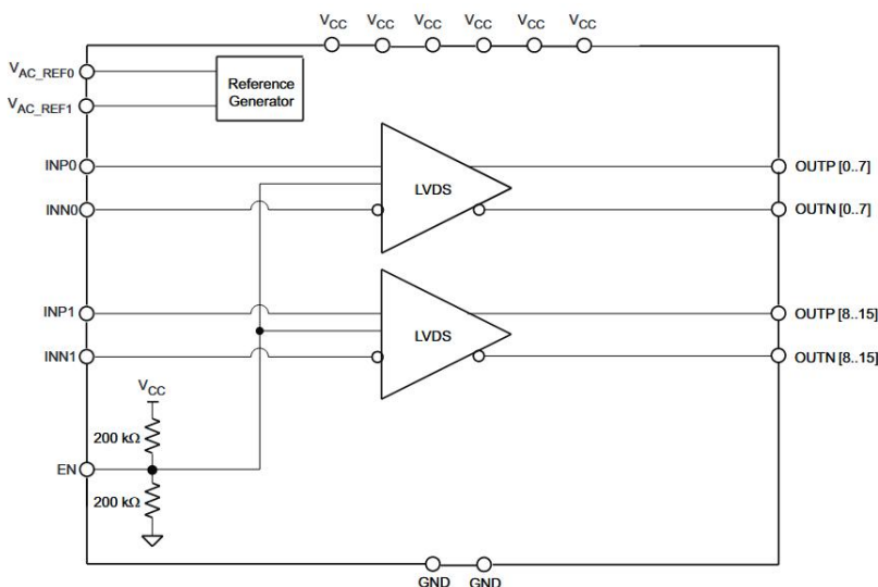
功能框图
