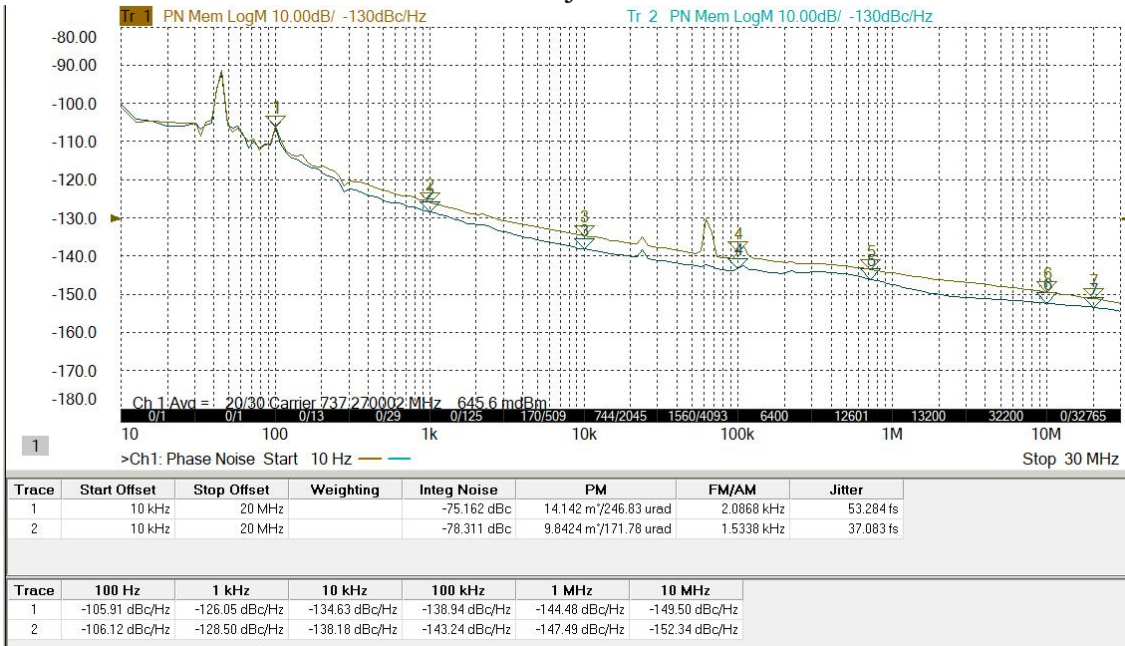
图 MBUFLVD2108在100MHz时相位噪声曲线
