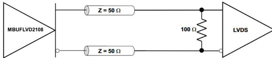
图 LVDS输出DC耦合连接
