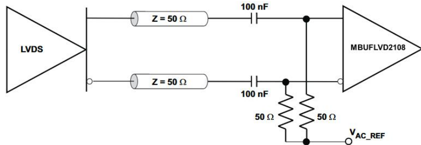
图 LVDS时钟驱动器连接到MBUFLVD2108输入（AC耦合）
