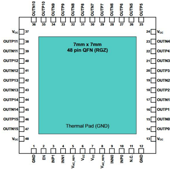
图 MBUFLVD2108引脚配置图
